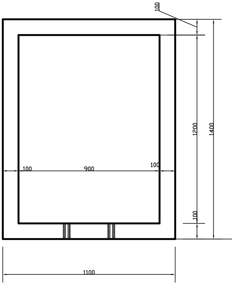
Podorys vodomernej šachty
